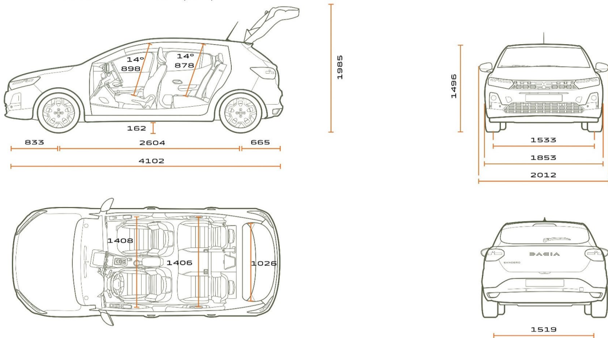
Διαστάσεις σε mm
